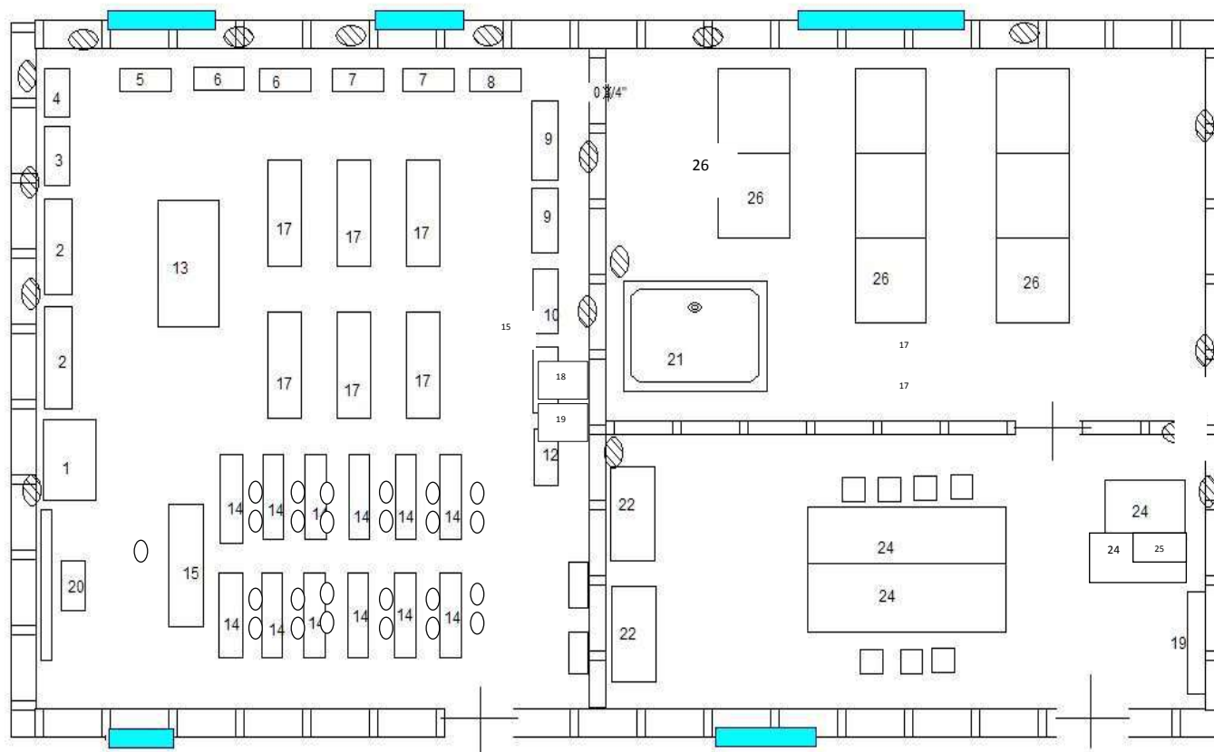
План застройки мастерской 3 по компетенции Сити-фермерство
